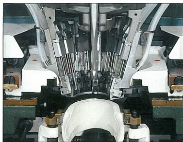
Plastre con posizione programmabile in apertura-chiusura e destro-sinistro Wipers with programmable position opening-closing and left-right Placas de montaje con posición programable en abertura-cierre y derecho-izquierdo 可程序调整张开大小及左右位置的扫刀
